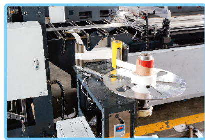
卡头纸放料架 Tyvek header paper feeding device
